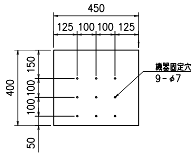
中間棚詳細
