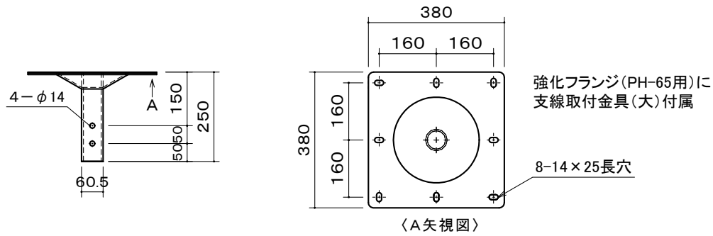
〈A矢視図〉
