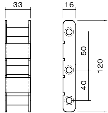
ジョイント金具
